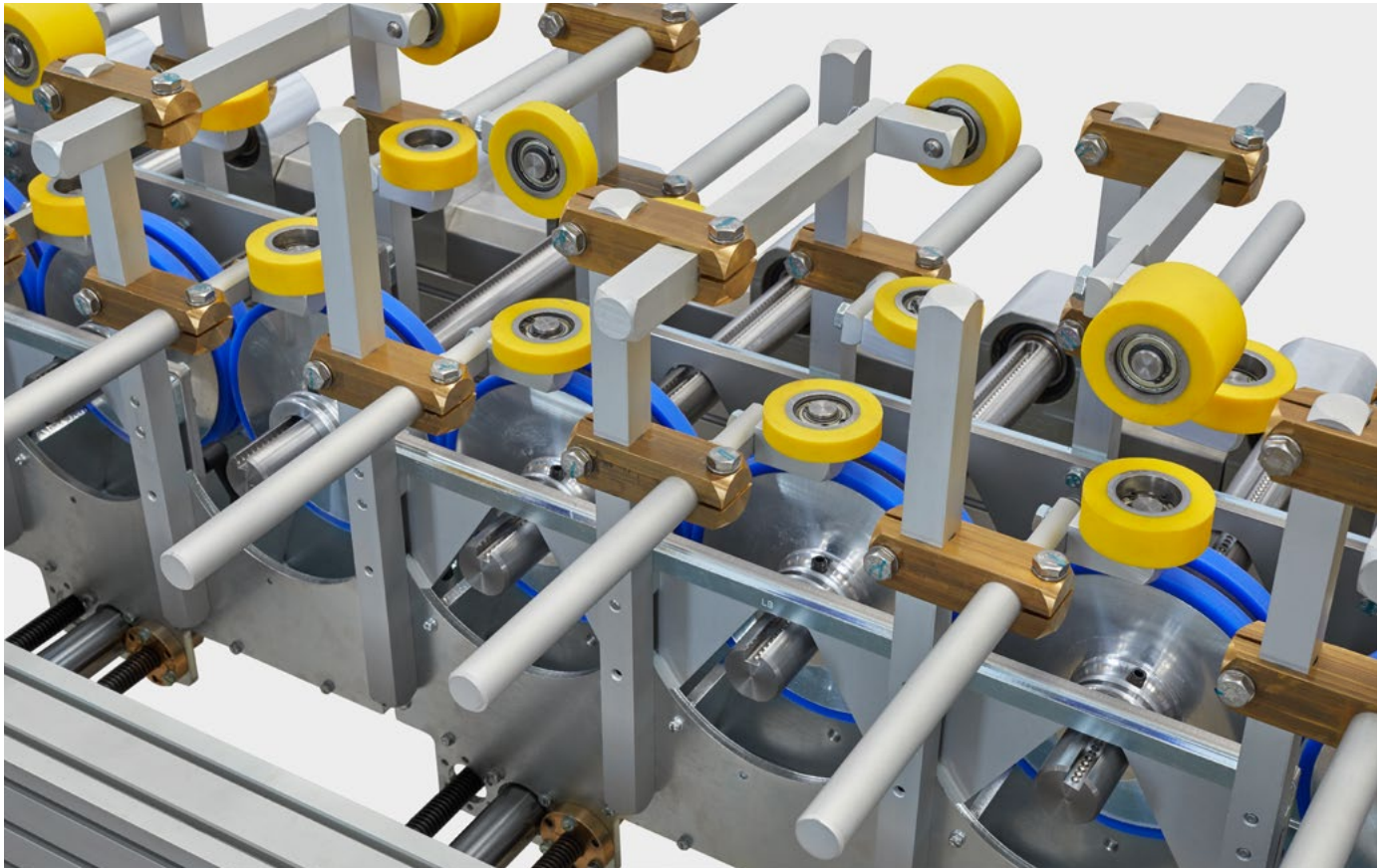
BILD: Ummantelungszone mit Quick-fix-System und Rasterverstellung der Transporträder
